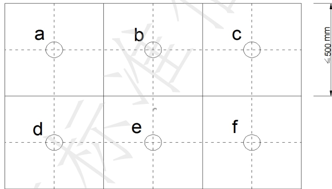
图 2 隔声涂料试件均分区域的测点位置
